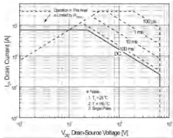
图 6-2 SIF7N65F(TO-220FP(L)) 最大安全工作区曲线 Fig6-2 Maximum Safe Operating Area
